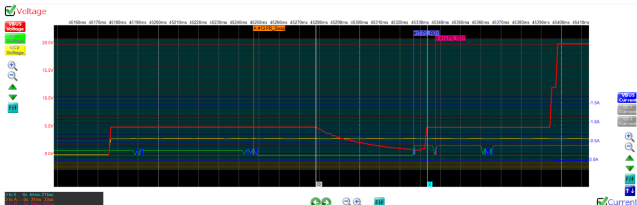
PR_SwapメッセージとVBUS電圧変化の測定例
